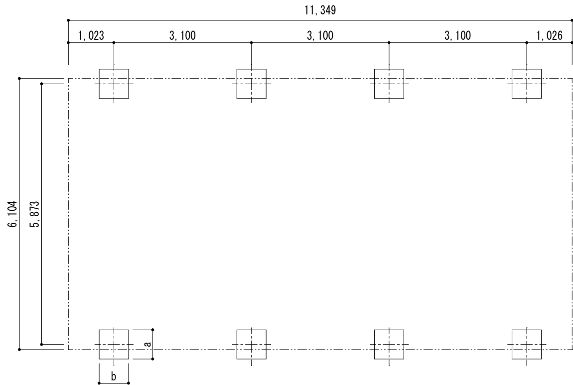
■基礎配置図
